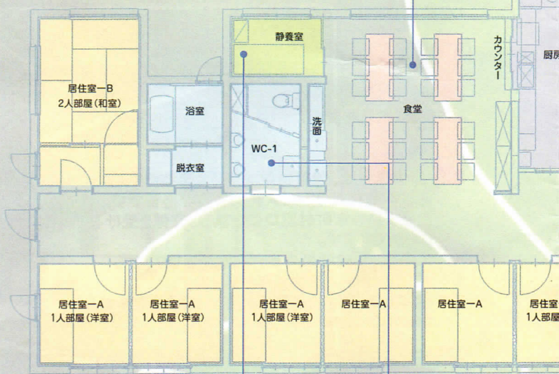
1階平面
